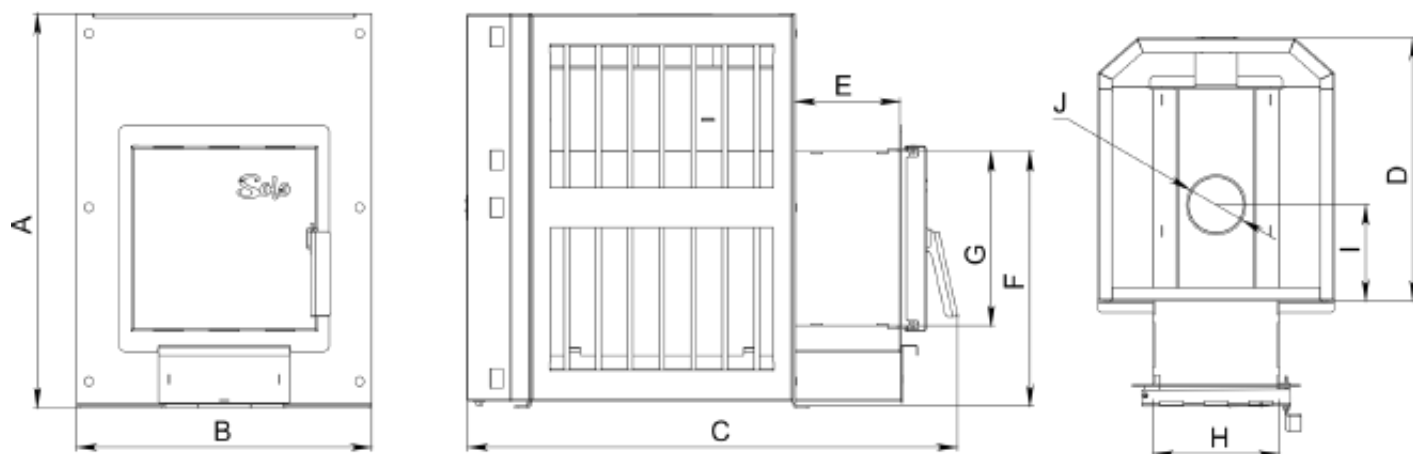
Рис. 2.1 Основные размеры печи SOLO(S)
